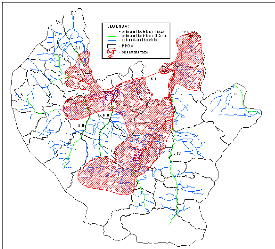
Slika 1 Situacioni prikaz 1. faze
